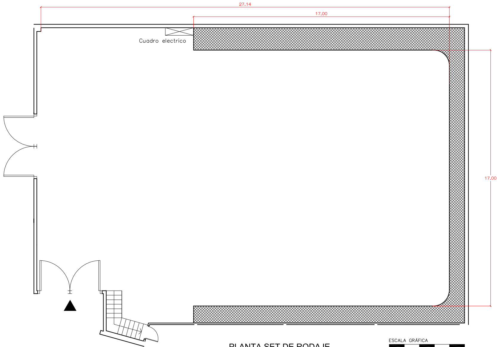
PLANTA SET DE RODAJE ESCALA 1:150
